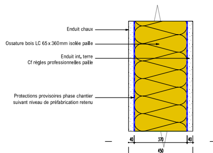
Coupe verticale MOB enduit. Carnet de détails, Bureau d'études Q.S.B.
