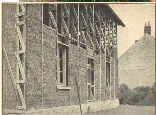
LES MURS DE LA MAISON ISOTHERMIQUE COMMENCENT À PRENDRE TOURNEUR Les blocs de paille comprimée sont superposés entre les montants de bois dont ils occupent toute l'épaisseur.
