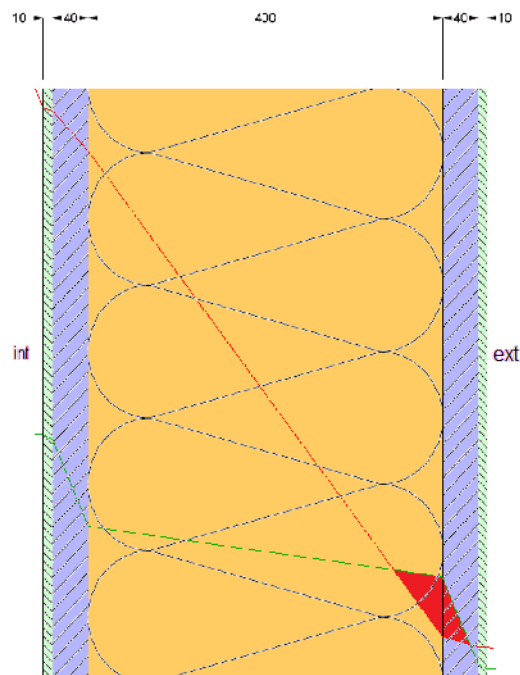
101 Coupe d'un mur en paille (technique GREB).
