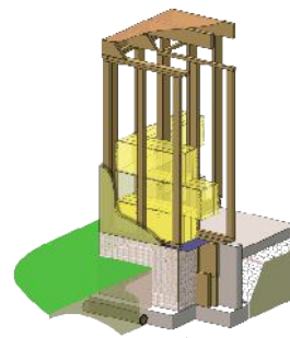
47 Schématisation et modélisation graphique d'un mur « technique GREB »
