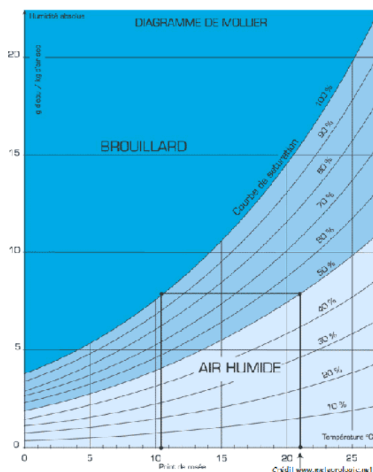
81 Diagramme de Mollier - courbe de l'air humide
