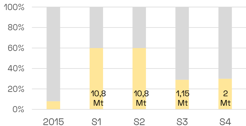
Parts (et volumes) d'isolants biosourcés en rénovation énergétique des logements de 2015 à 2050 – Source données : Ademe Transition(s) 2050
